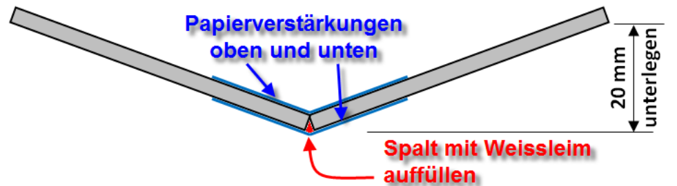
Längsschnitt Leitwerk 1:1
