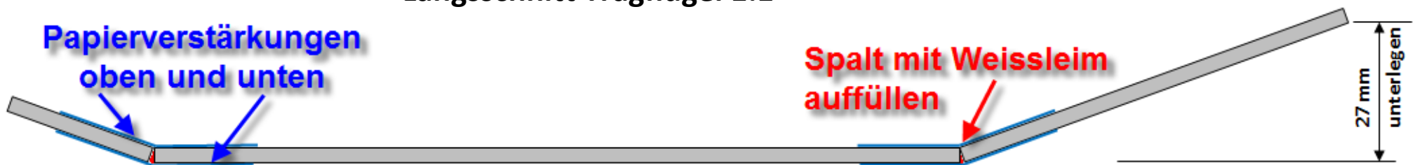
Längsschnitt Tragflügel 1:1
